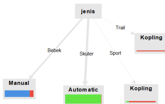
Gambar 1. Pohon Keputusan
